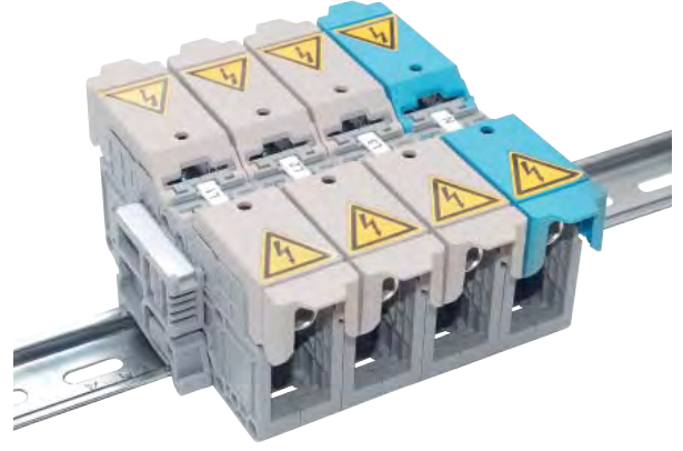
MRK SERİSİ PAPUÇ BAĞLANTILI BARALI RAY KLEMENSLER (KAPAKLI)
