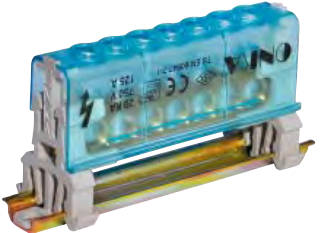
Kablo kesiti max. 25 mm 2 (Yüksüklü) - 35 mm 2 (Yüksüksüz)
