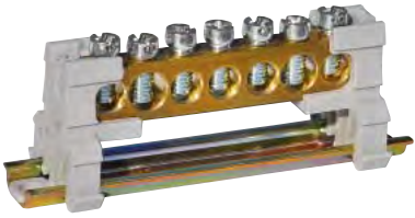
Kablo kesiti max. 25 mm 2 (Yüksüklü) - 35 mm 2 (Yüksüksüz)
