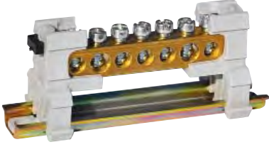
Kablo kesiti max. 10 mm 2 (Yüksüklü) - 16 mm 2 (Yüksüksüz)
