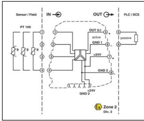
MINI MCR-SL-PT 100-UI... için bağlantı şekli
