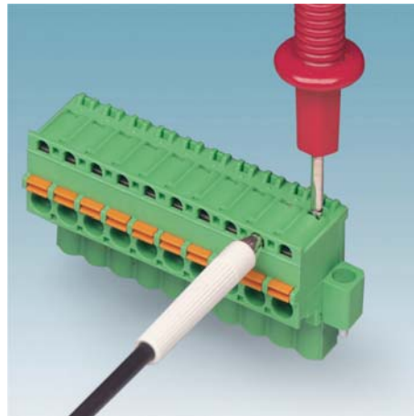
Entegre test bağlantıları
