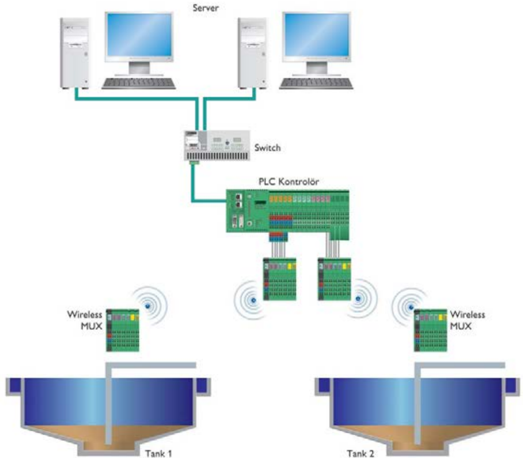
MUX için bağlantı şeması
