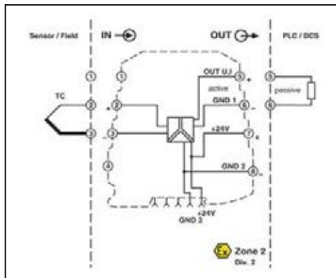
MINI MCR-SL-TC-UI-NC için bağlantı şekli
