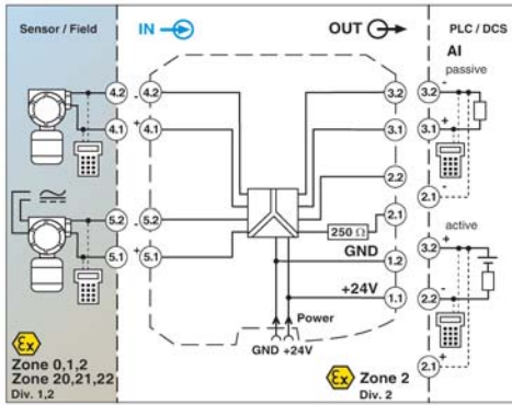
MACX MCR-EX-SL-RPSSI-I için bağlantı şekli
