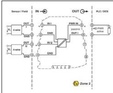
MINI MCR-SL-UI-I-LP-NC için bağlantı şekli
