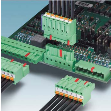
Aynı kutup sayısındaki konnektörlerin yanlış takılmasını önler
