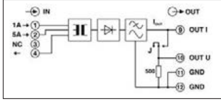
MCR-SLP-1-5-UI-0 bağlantı şekli
