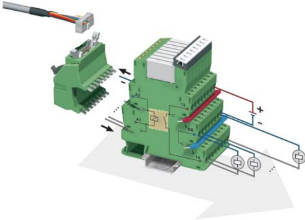
Aktüatör serisi röle uygulama resmi.
