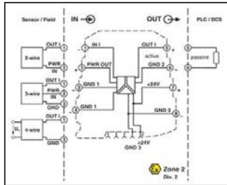
MINI MCR-SL-RPS-I-I için bağlantı şekli
