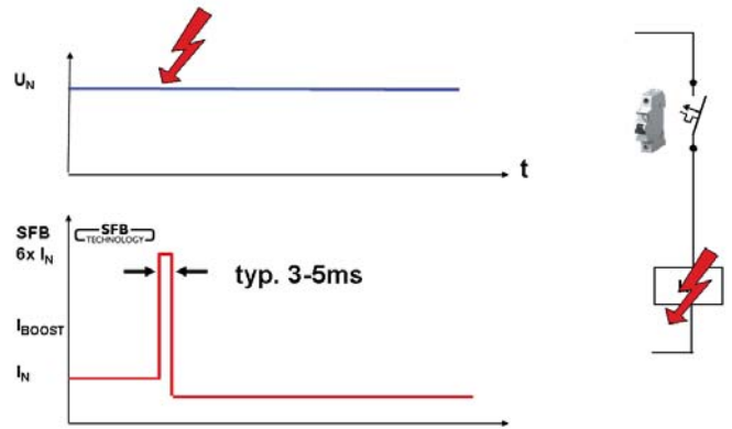
Sigorta attırma özelliği
