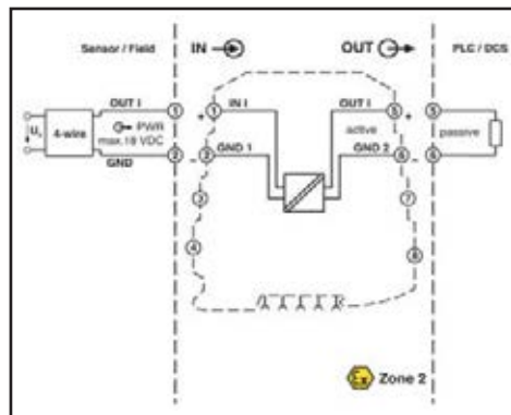
MINI MCR-SL-1CP-I-I için bağlantı şekli
