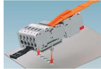
COMBI soketlerin pinlerle saca monte edilebilen tipleri de bulunmaktadır
