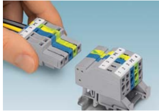
Raya montaj ayaklı soket uygulaması NS 35 ve NS 15 raylar için uygundur
