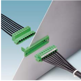
DFK-MSTBA 2,5/...-G-5,08 +MSTB 2,5/...-5,08
