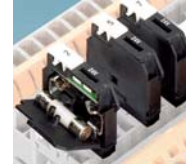
P-FU sigorta fişleri ayırma kolları sigortalı klemenslerin alternatifidir
