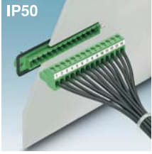
DFK-MSTBA 2,5/...-G-5,08 +MSTB 2,5/...-5,08
