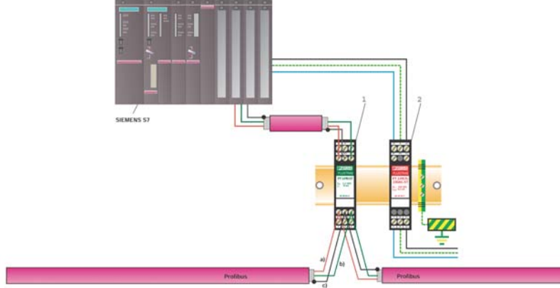
PROFIBUS KORUMA BAĞLANTI ŞEMASI
