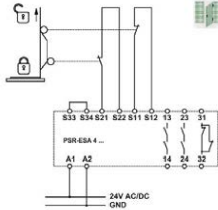
2963750 Örnek bağlantı şeması 2 kanal emniyet kapısı izleme, otomatik aktivasyon özelliği vardır. Kategori 4'e uygundur.
