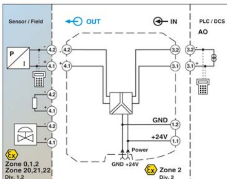
MACX MCR-EX-SL-IDSI-I için bağlantı şekli
