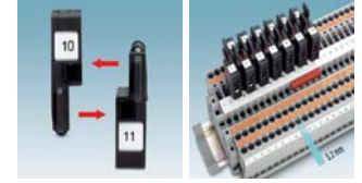
P-FU ...-5 sigorta fişi 5,2 mm genişlikte (2,5 mm 2 'lik) ...TG ayırma klemensleriyle kullanılabilir ve maksimum alan kazancı sağlar.
