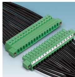
Havada bağlantı flanşlı fiş ve evrik fiş IMC 1,5/...-STF-3,81 & MC 1,5/...-ST-3,81
