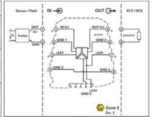
MINI MCR-SL-UI-UI-NC için bağlantı şekli
