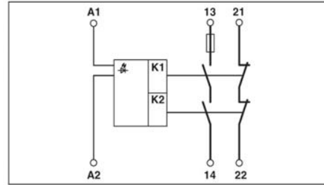
2981978 Örnek bağlantı şeması
