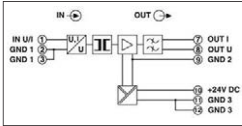
MCR-C-UI-UI-DCI-NC için bağlantı şekli
