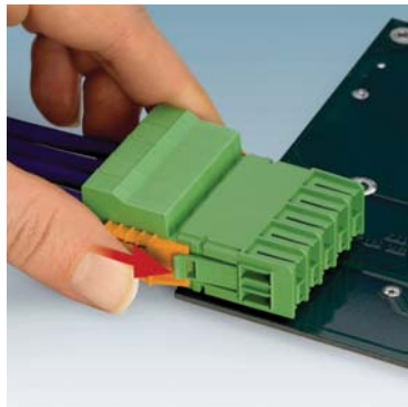
PC5: CLICK & LOCK sisteminde fiş soketten iki basit hareket ile ayrılabilir
