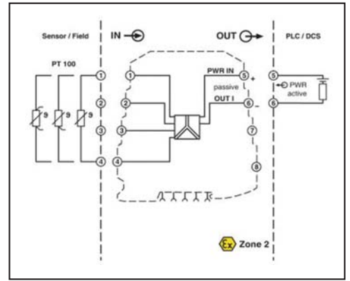
MINI MCR-SL-PT100-LP-NC için bağlantı şekli
