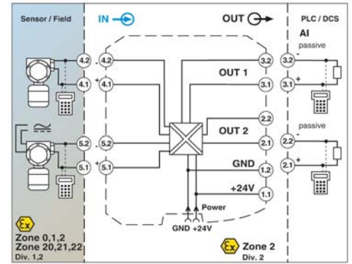
MACX MCR-EX-SL-RPSSI-2I için bağlantı şekli
