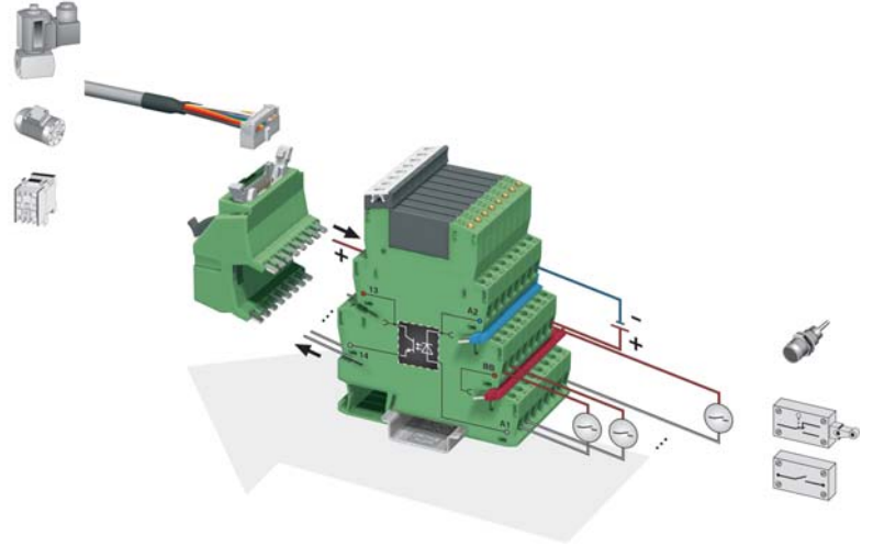
Sensör serisi röle uygulama resmi.
