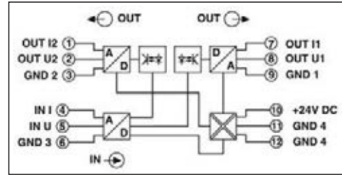
MCR-FL-C-UI-2UI-DCI-NC için bağlantı şekli
