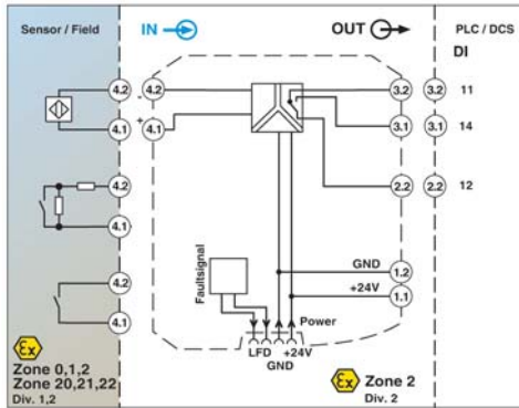
MACX MCR-EX-SL-NAM-R için bağlantı şekilleri
