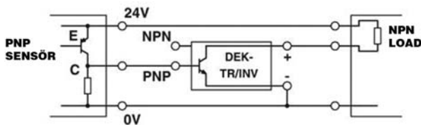
DEK-TR/INV bağlantı şekilleri
