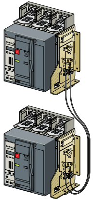
Kablo ile dikey mekanik kilitleme
