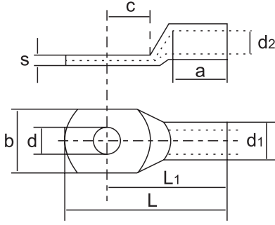
SIKMALI KABLO PABUÇLARI (SKP) COMPRESSIVE CABLE LUGS
